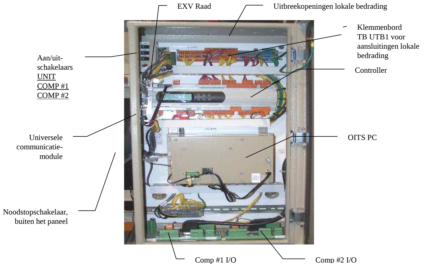
Afbeelding 2, Regelpaneel
