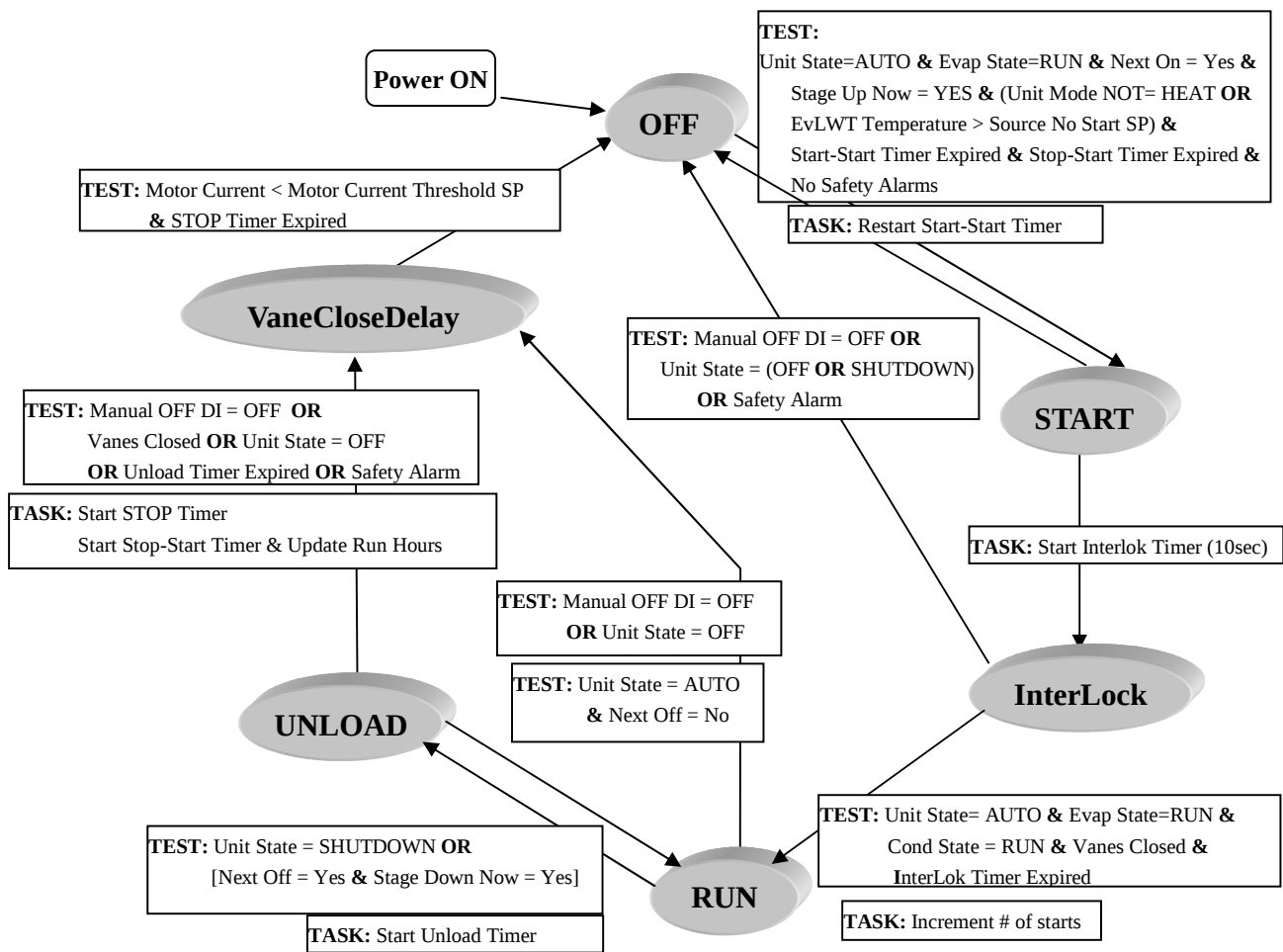
Afbeelding 6, Compressorstaat
