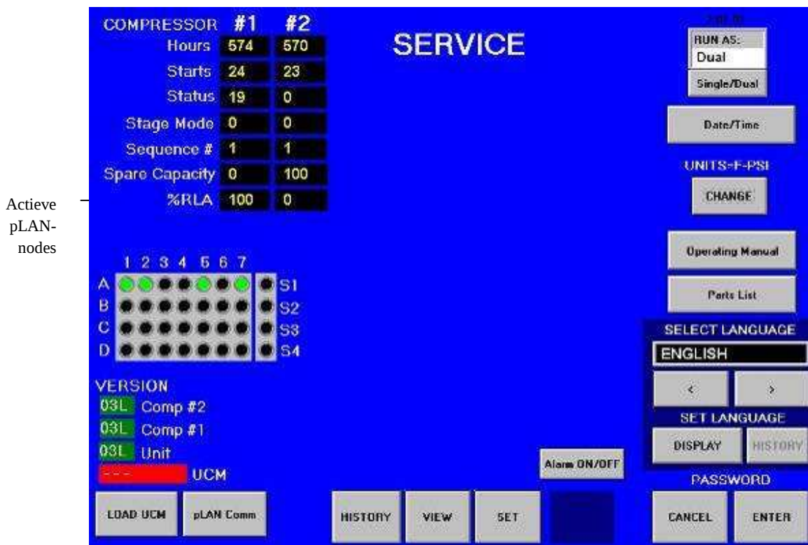
Afbeelding 26, Scherm Service
