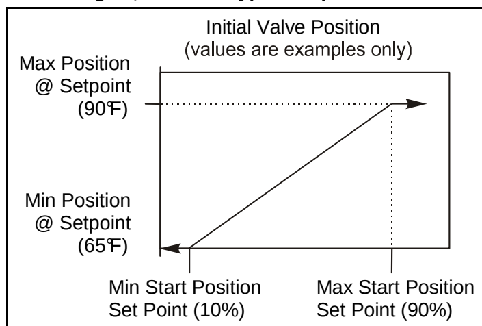
Afbeelding 22, Standen bypassklep
