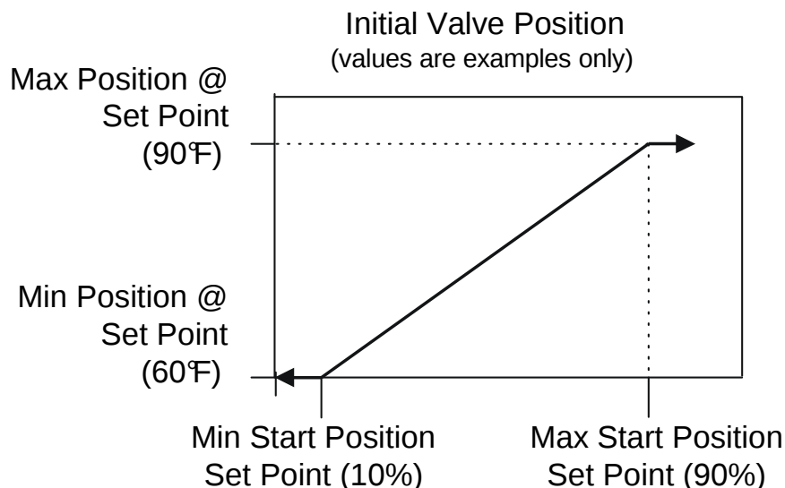
Afbeelding 32, Stand bypassklep
