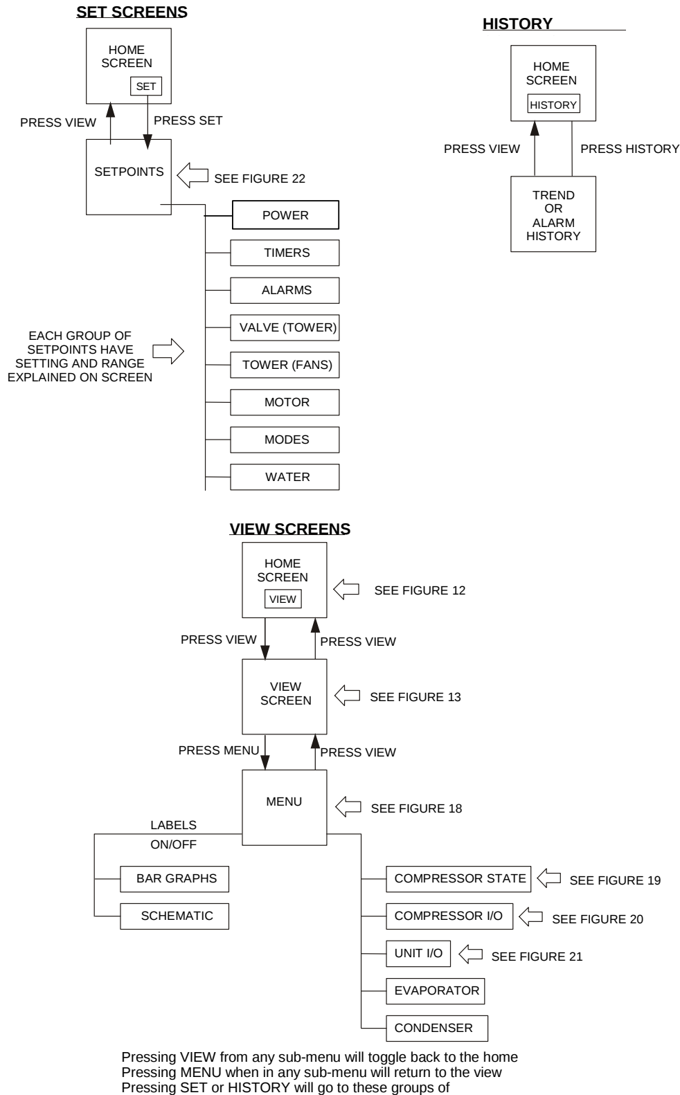
Afbeelding 9, schermlayout aanraakscherm
