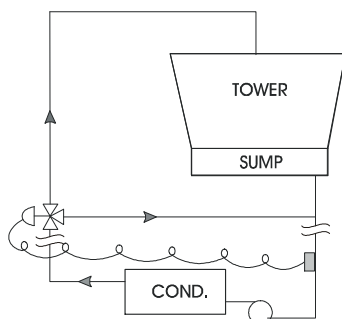
Afbeelding 3, Bypass, werking bij zacht weer
