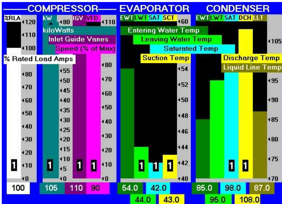
Afbeelding 16, Gelabelde staafdiagrammen
