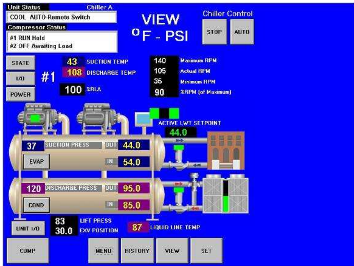
Afbeelding 11, Detail View-schermb
