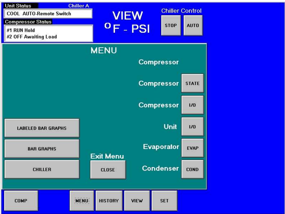
Afbeelding 12, Menu View
