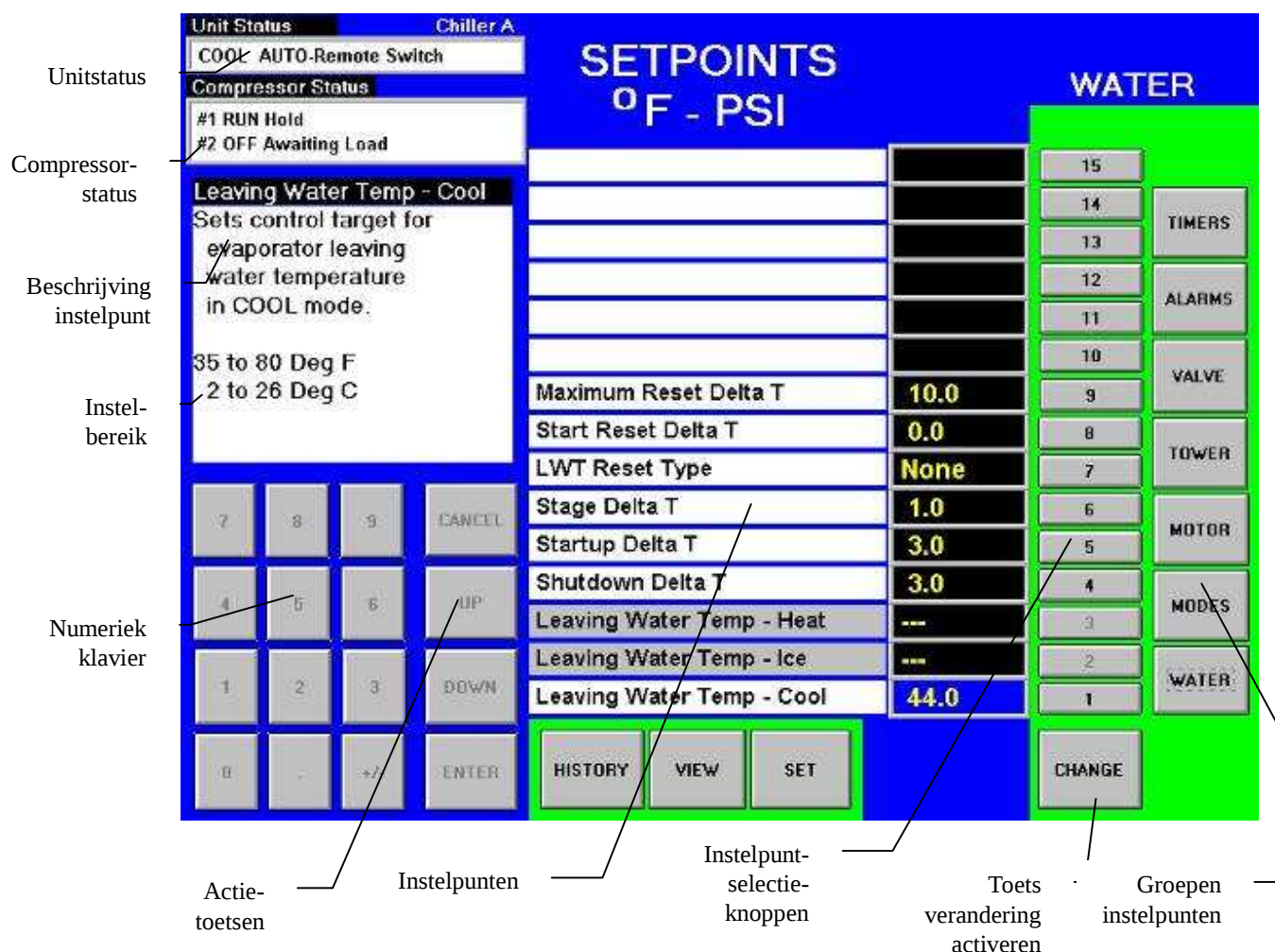
Afbeelding 17, Typisch SETPOINT-scherm
