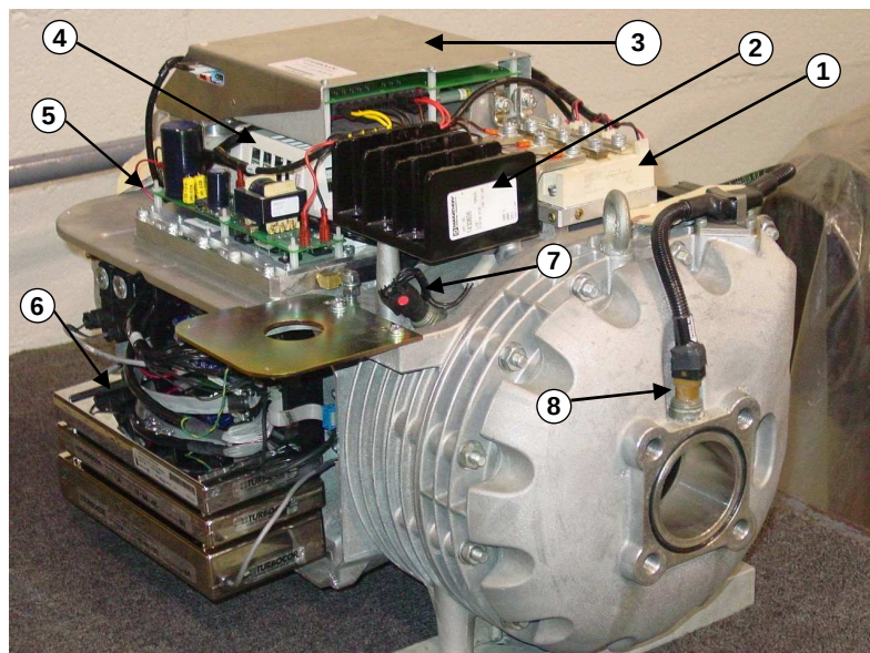
Afbeelding 7, Elektrische/Elektronische componenten compressor
