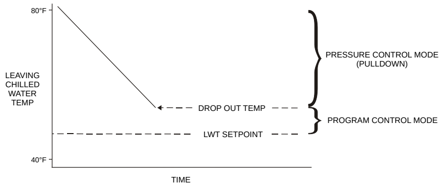
Afbeelding 31, Wegvallen drukregeling
