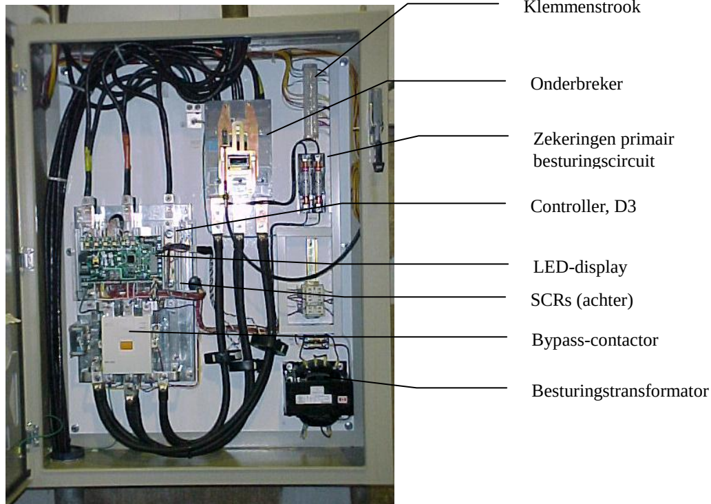
Afbeelding 37, Solid State starter, wandmontage
