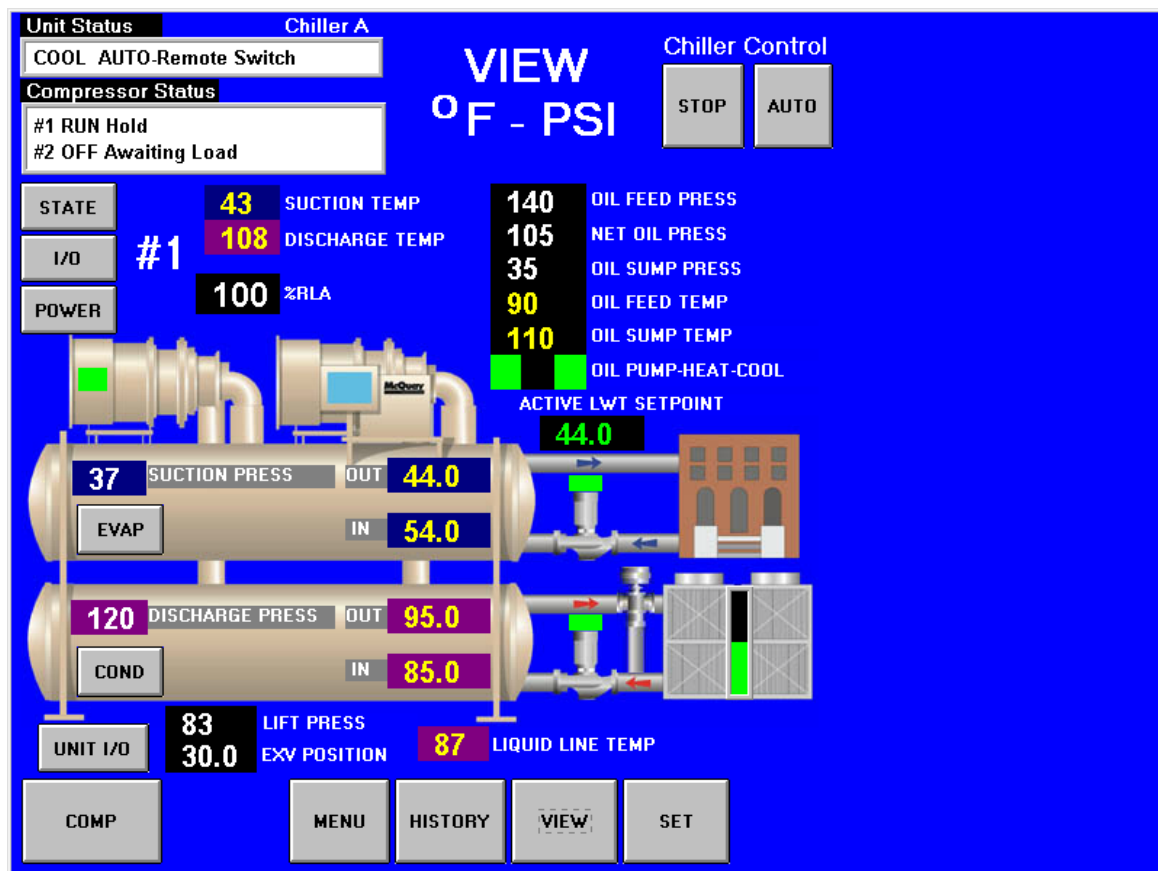
Afbeelding 6, Detail View-scherm
