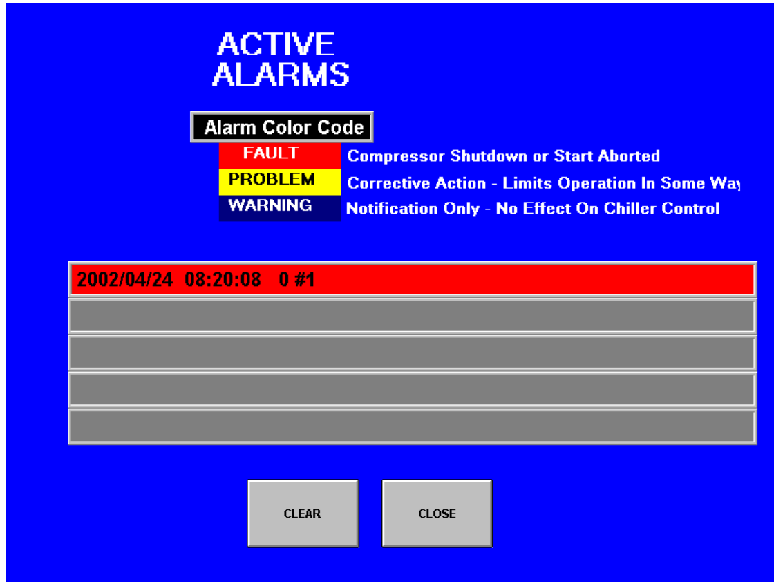
Afbeelding 25, Active Alarms
