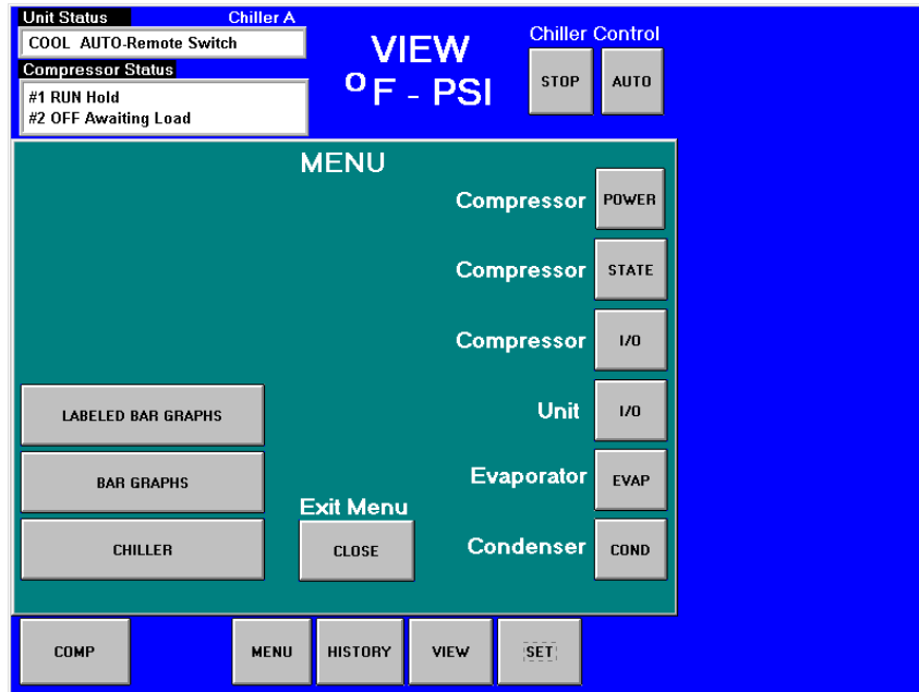
Afbeelding 8, Menu View
