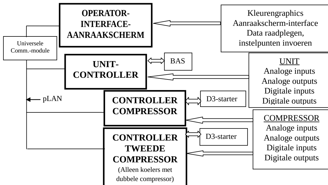
Afbeelding 1, Voornaamste besturingscomponenten
