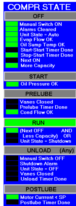
Afbeelding 9, Scherm View Compressor State
