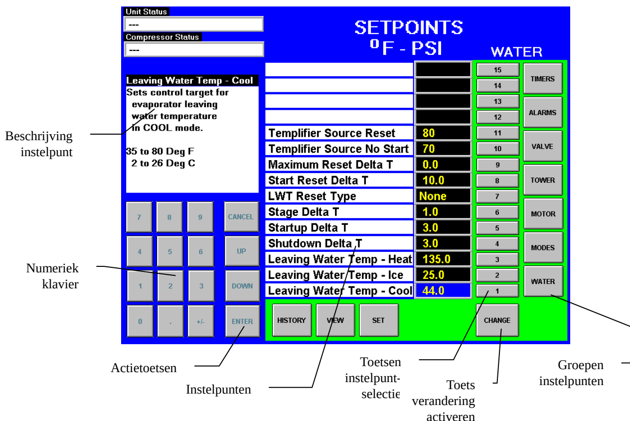
Afbeelding 13, Typisch SETPOINT-scherm
