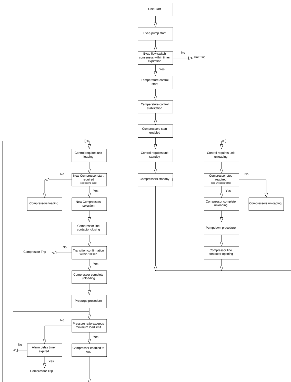
Afbeelding 17 – Opstartsequentie unit
