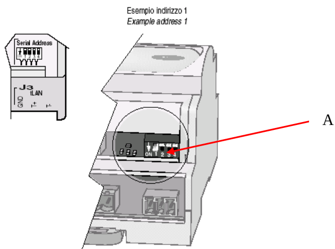
Afbeelding 6 – pCO e detail: schakelaars
