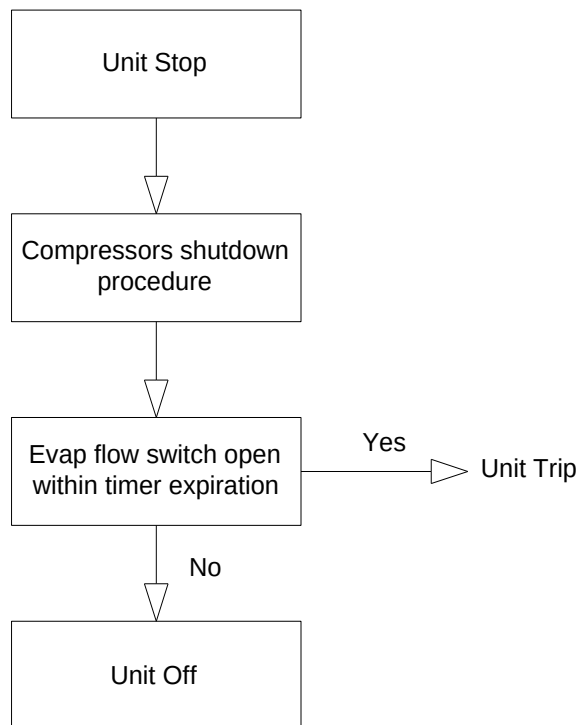
Afbeelding 18 – Uitschakelsequentie unit
