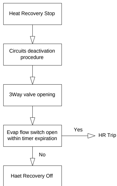
Afbeelding 20 – Uitschakelsequentie warmteterugwinning
