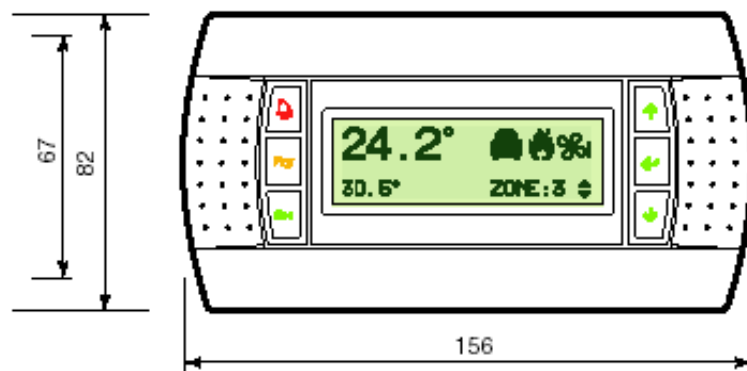
Afbeelding 3 – PGD-display
