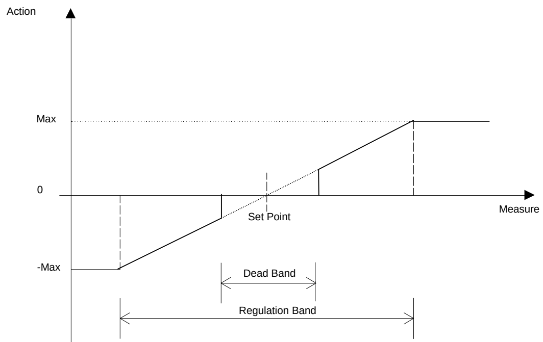
Afbeelding 12 – Proportionele actie PD-controller
