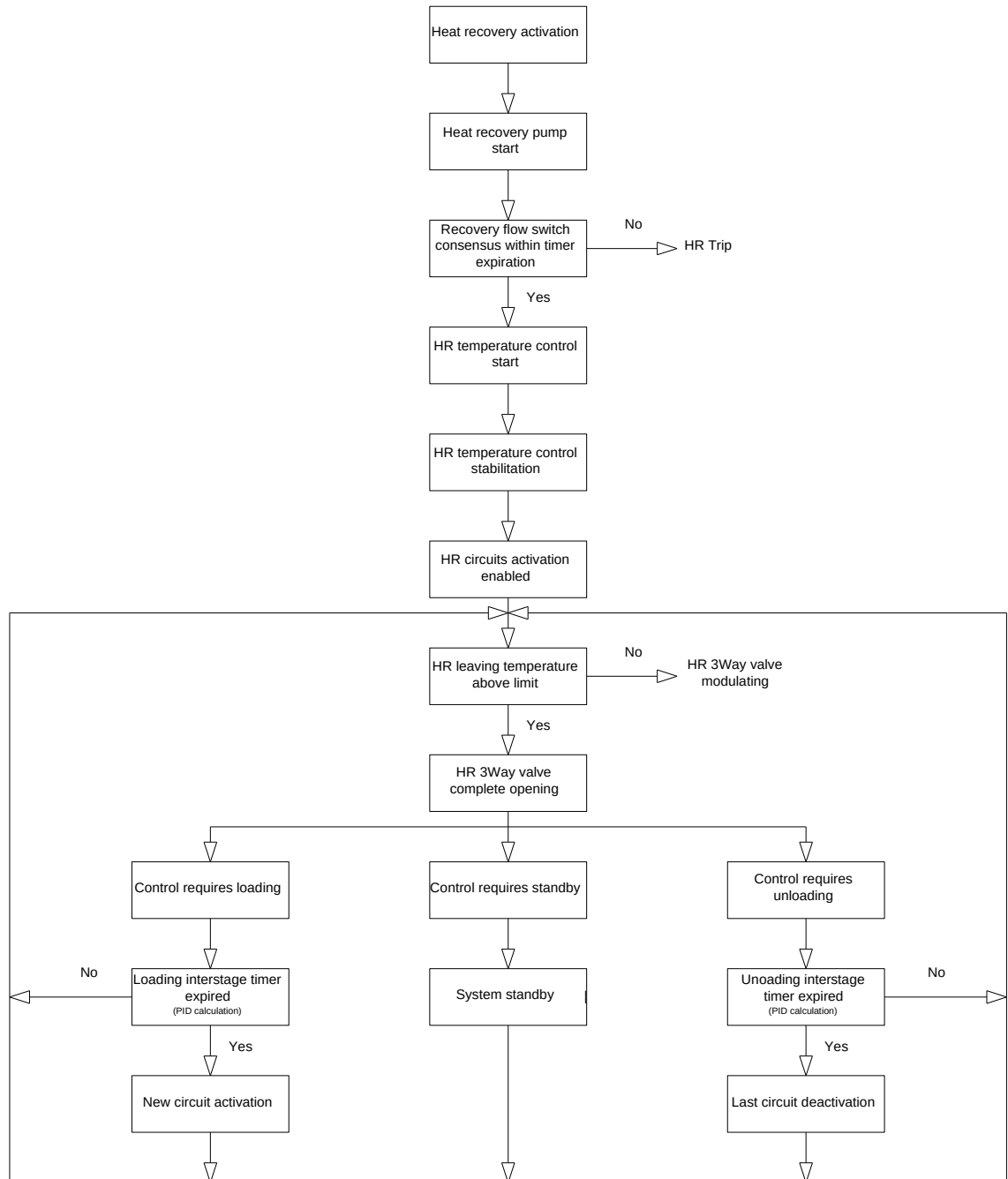
Afbeelding 19 – Opstartsequentie warmteterugwinning
