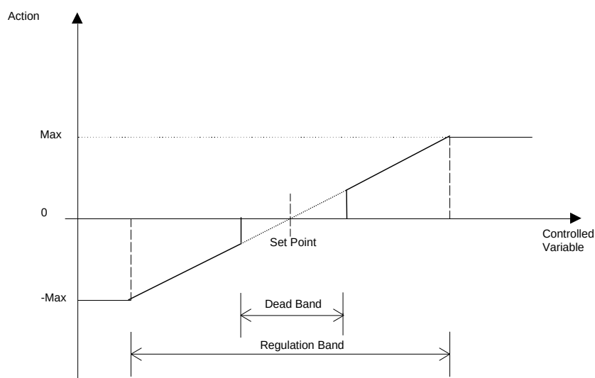
Afbeelding 15 – Proportionele actie van VSD PID in koelen/ijsstand
