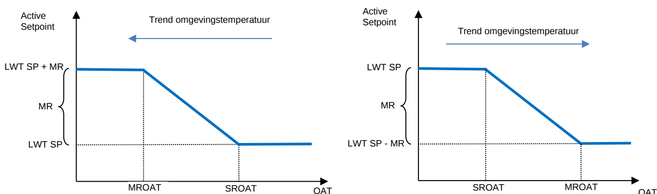
Grafiek 2 Omgevingstemperatuur tegen Active Setpoint – Cooling Mode (links) / Heating Mode (rechts)
