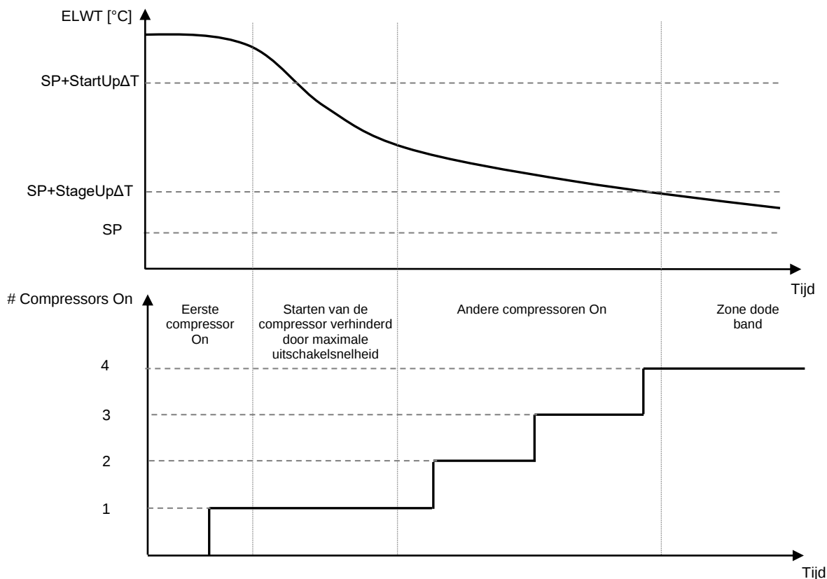
Opstartvolgorde compressoren - Modus Koelen
