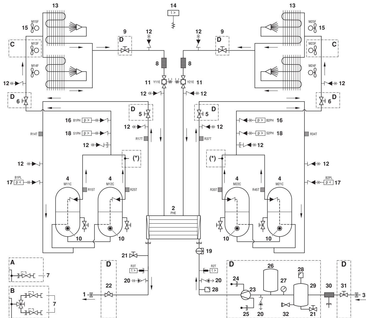
Afbeelding - Functioneel schema
