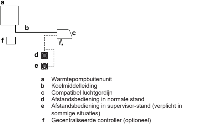
Aansluiting luchtgordijn
