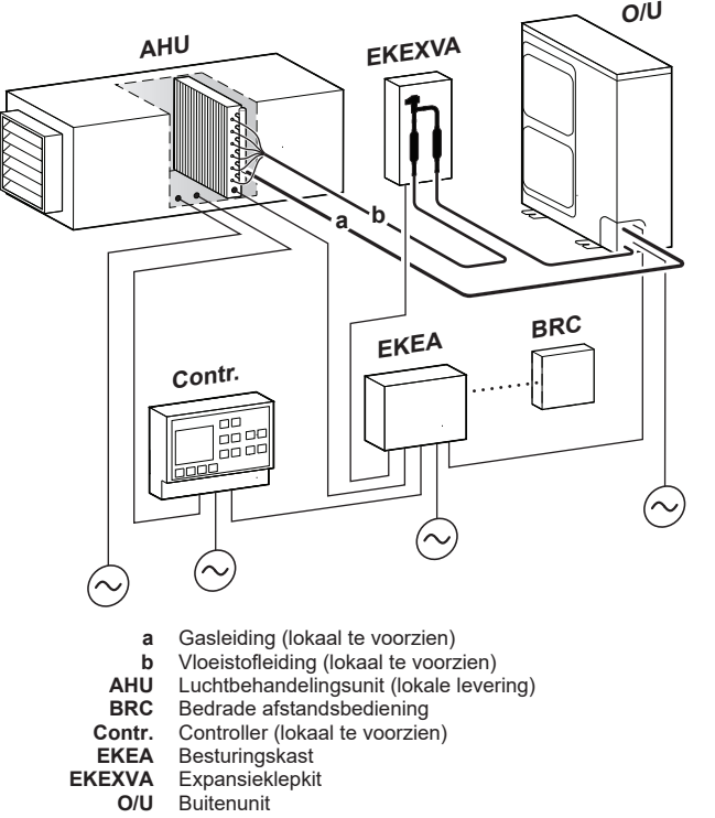
Aansluiting AHU
