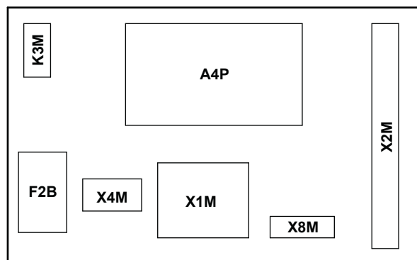
Plaats in de regelkast
