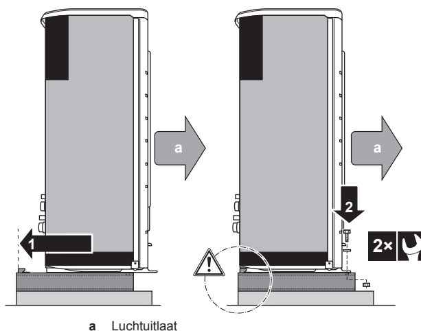
a Luchtuitlaat
