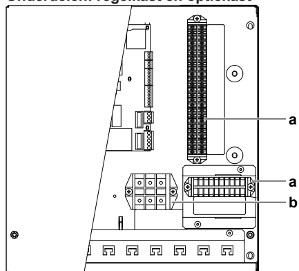
Onderdelen: regelkast en optiekast
