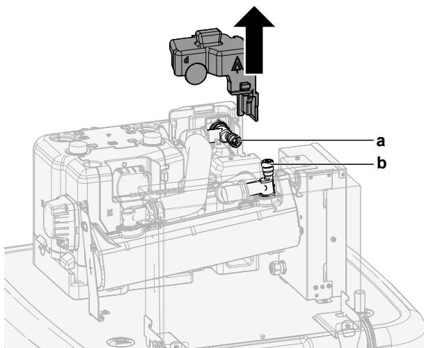
a, b Handbediende ontluhtingsklep
