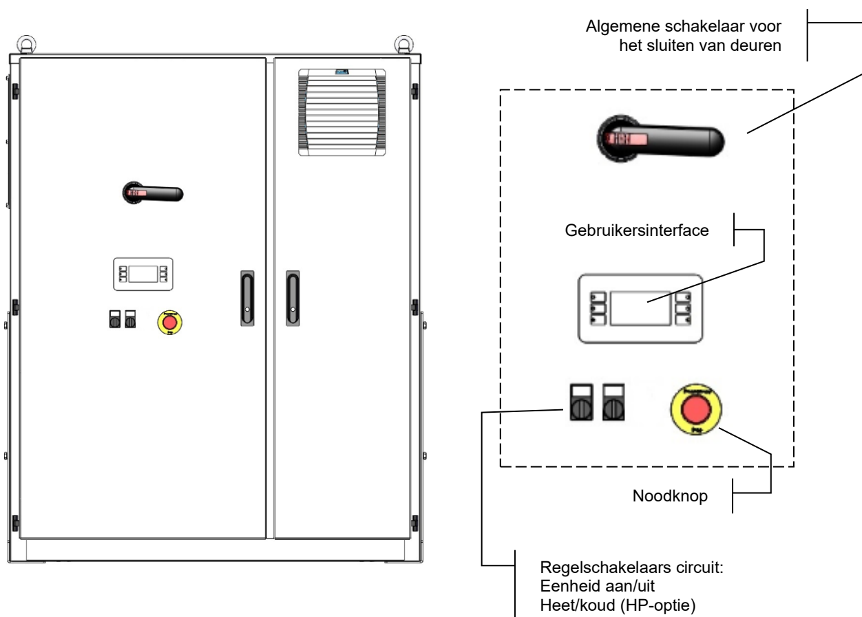
Afbeelding15 – Interface eenheid
