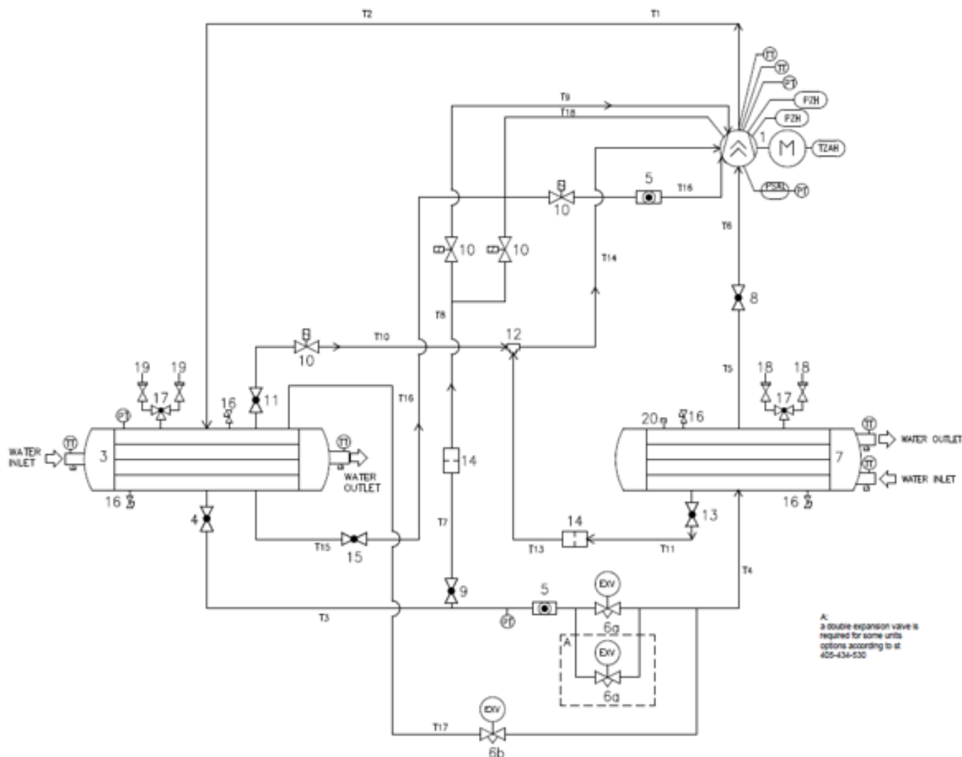
Afbeelding14 - P&ID optie251
