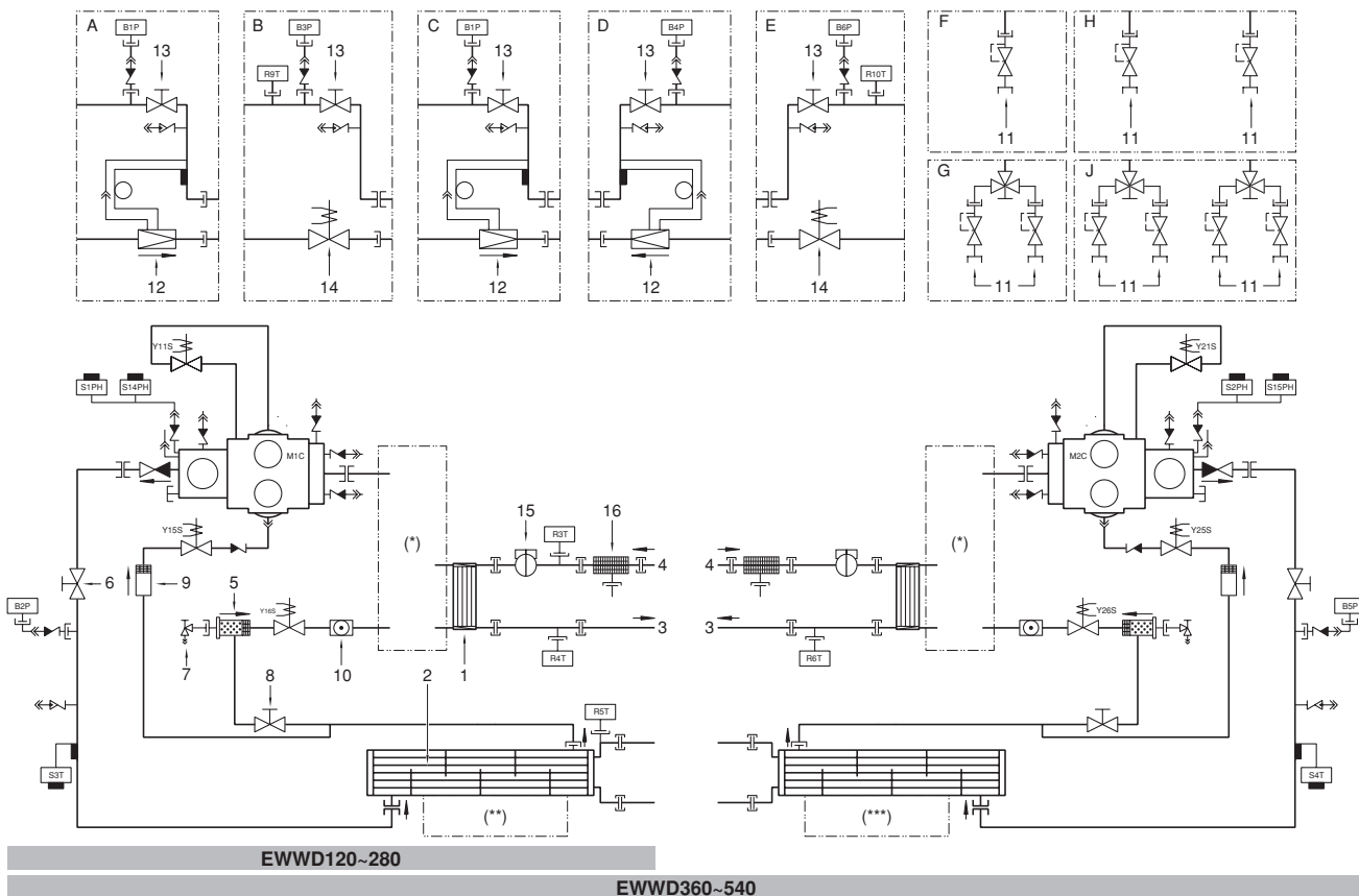
Afbeelding - Functioneel schema
