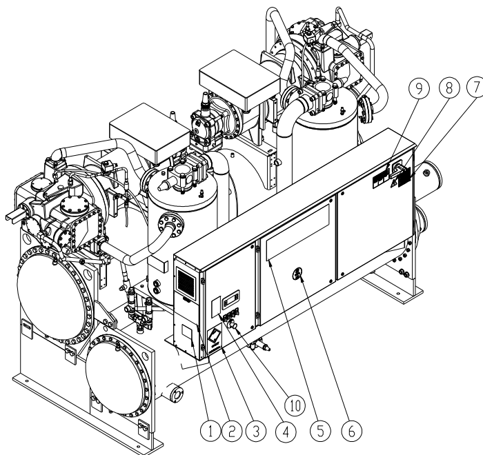
Jednostka z dwoma obiegami
