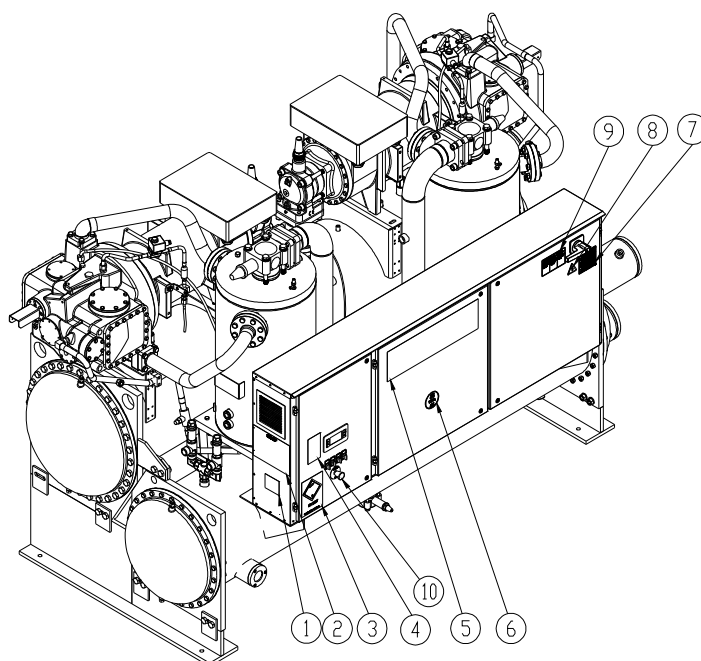
Einheit mit zwei Kühlkreisläufen
