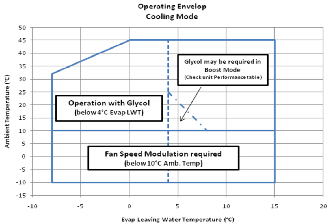
Afbeelding 1 - Bedrijfsbeperkingen in koelstand - EWYD-BZSS / EWYD-BZSL
