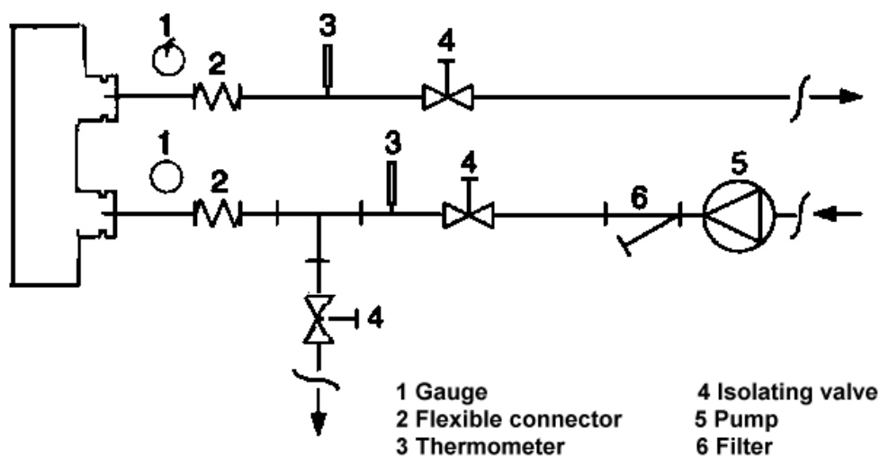
Afbeelding 6 - Waterleidingaansluiting voor verdamper
