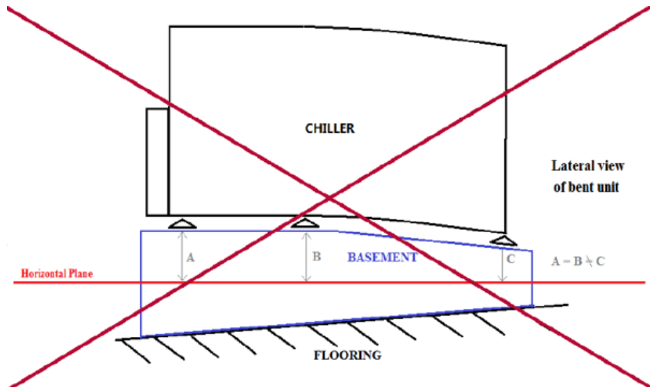
Afb. 13– Waterpasstelling systeem
