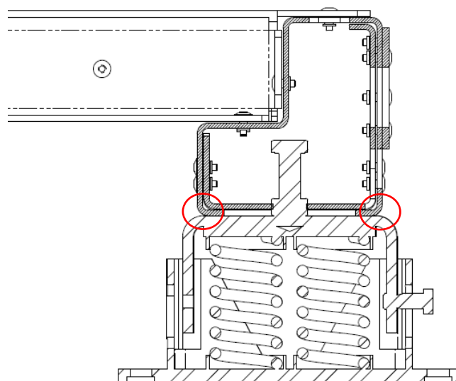
Afb. 18 - Antitrillingselementen monteren (geleverd als optie)
