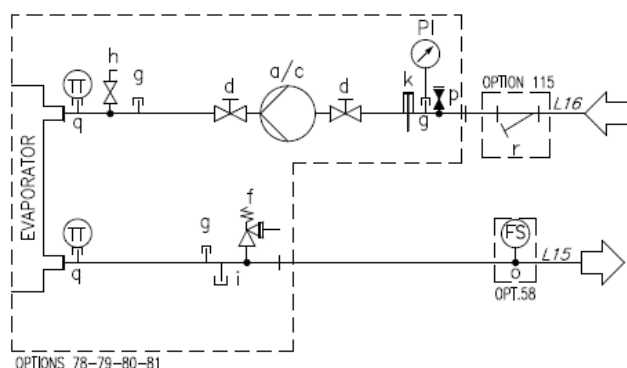
Afb. 19– Hydraulisch schema (opt. 78-79-80-81/134-135-136-137)
