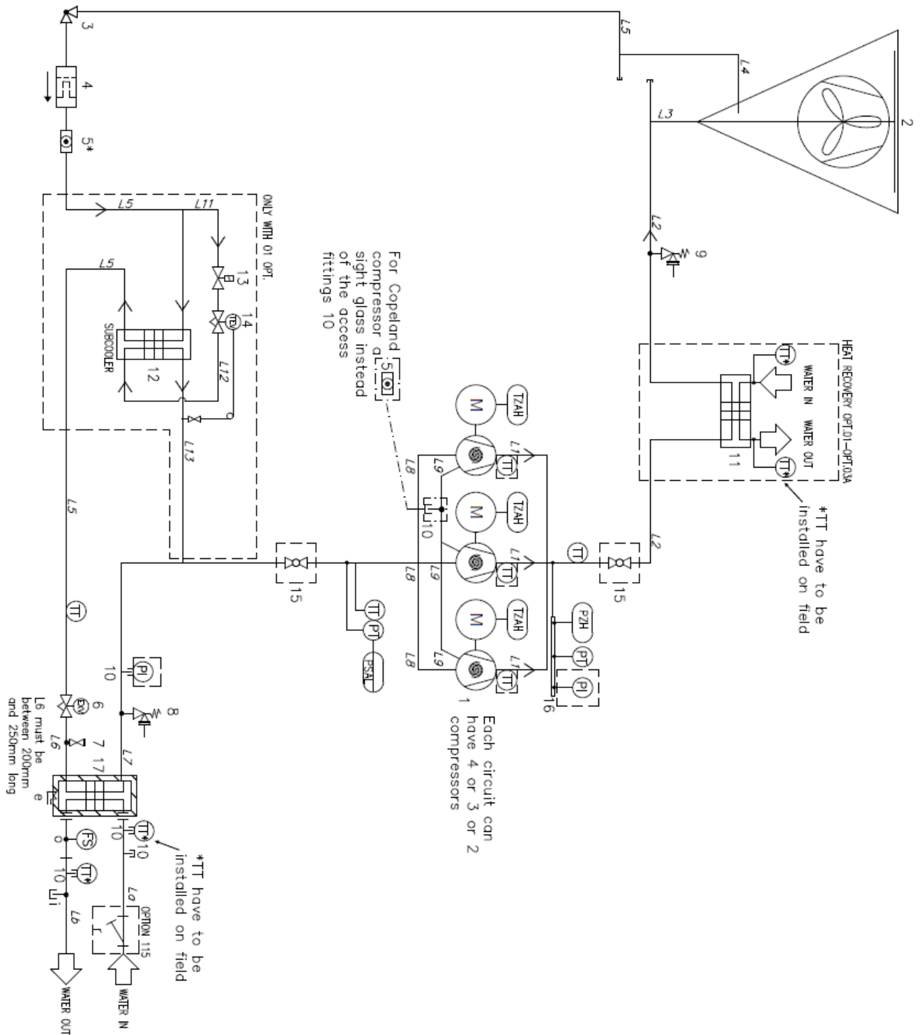
Afb. 1– Schema koelcircuit (P&ID) standaardsysteem met enkel circuit
