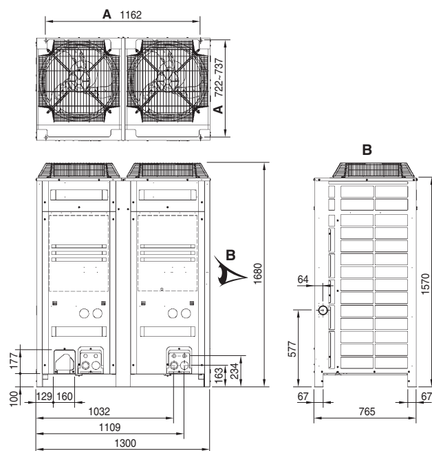
1 Afstanden van boutgaten onderstuk (15 x 22,5 langwerpige gaten)
