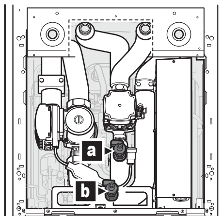
a Aftapkraan watercircuit b Aftapkraan pekeltcircuit
