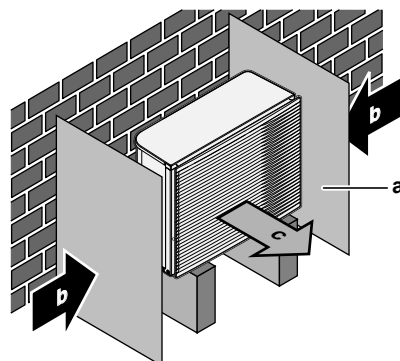
a Stootplaat
