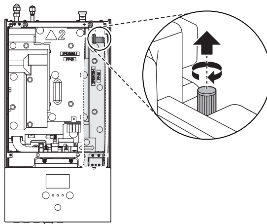
a Schrader-klep
