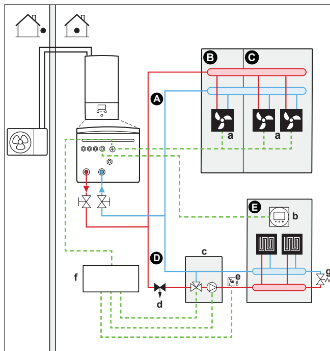
2 Systeem met hydraulische afscheider voor primaire zone:
