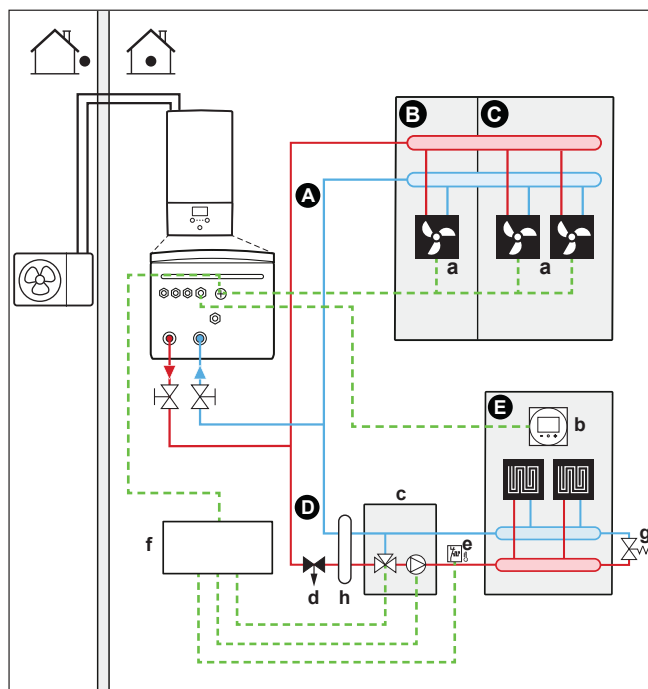
3 Systeem met hydraulische afscheider voor beide zones: Voor dit systeem is een directe pomp nodig voor de secundaire zone.
