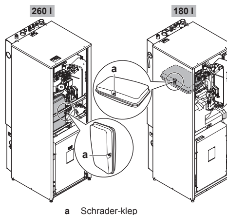
a Schrader-klep
