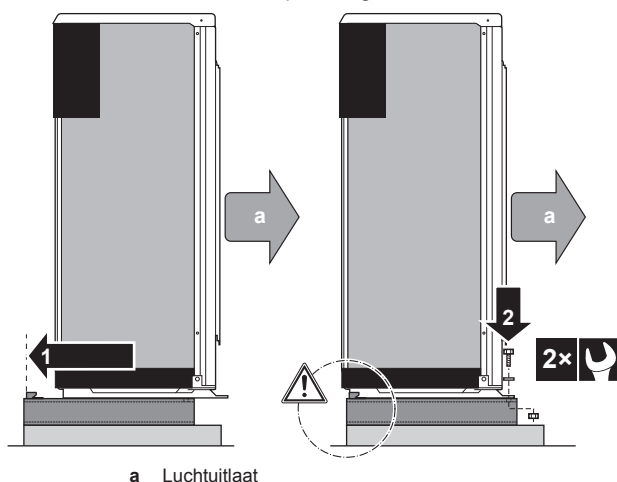
a Luchtuitlaat
