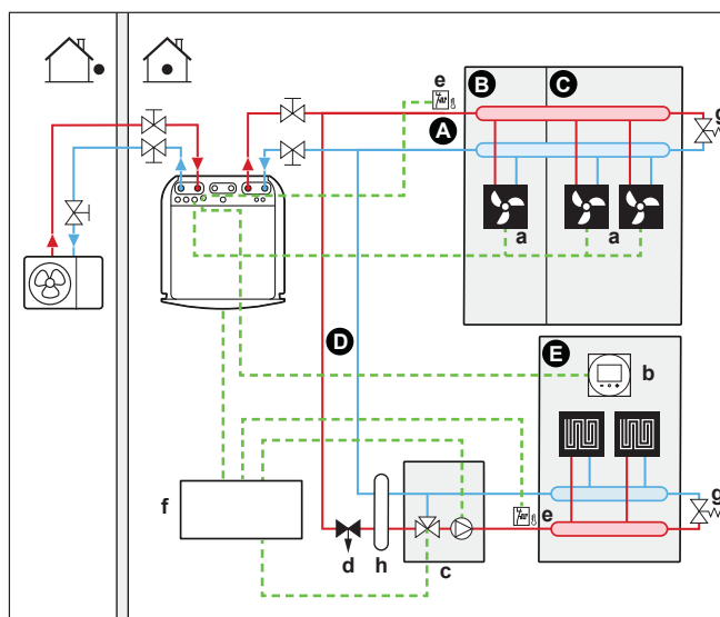
3 Systeem met hydraulische afscheider voor beide zones: Voor dit systeem is een directe pomp nodig voor de secundaire zone.
