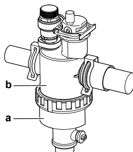
a Onderste gedeelte dat moet worden losgeschroefd
