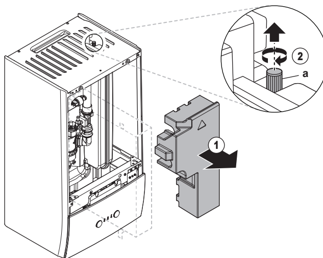
a Schrader-klep
