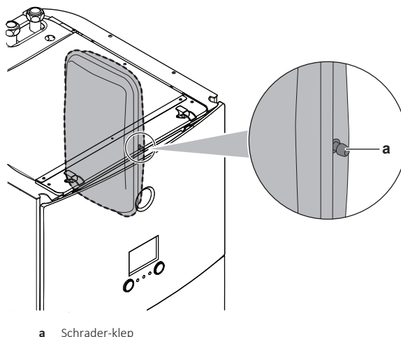
a Schrader-klep
