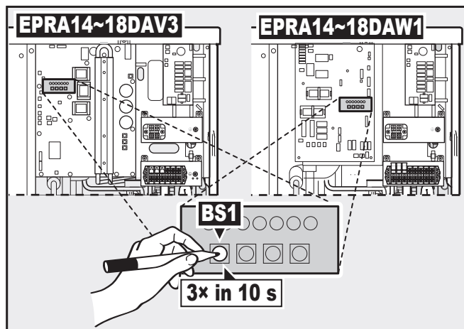
a Drukknop
