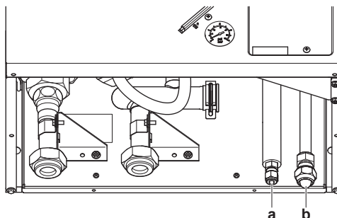
a Aansluiting voor de koelvloeistof b Aansluiting voor het koelgas
