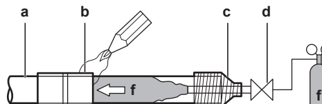
a Koelmiddelleiding b Te hardsolderen deel c Tape d Handbediende klep e Reduceerklep f Stikstof
