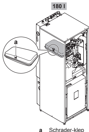
a Schrader-klep
