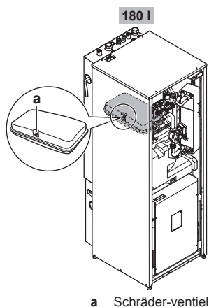
a Schröder-ventiel
