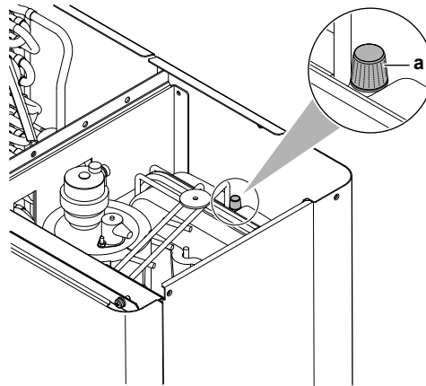
a Schrader-klep
