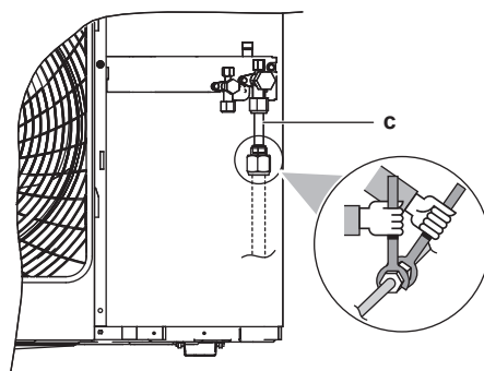
c Gasleidingaccessoire (alleen voor RXYSCQ6)
