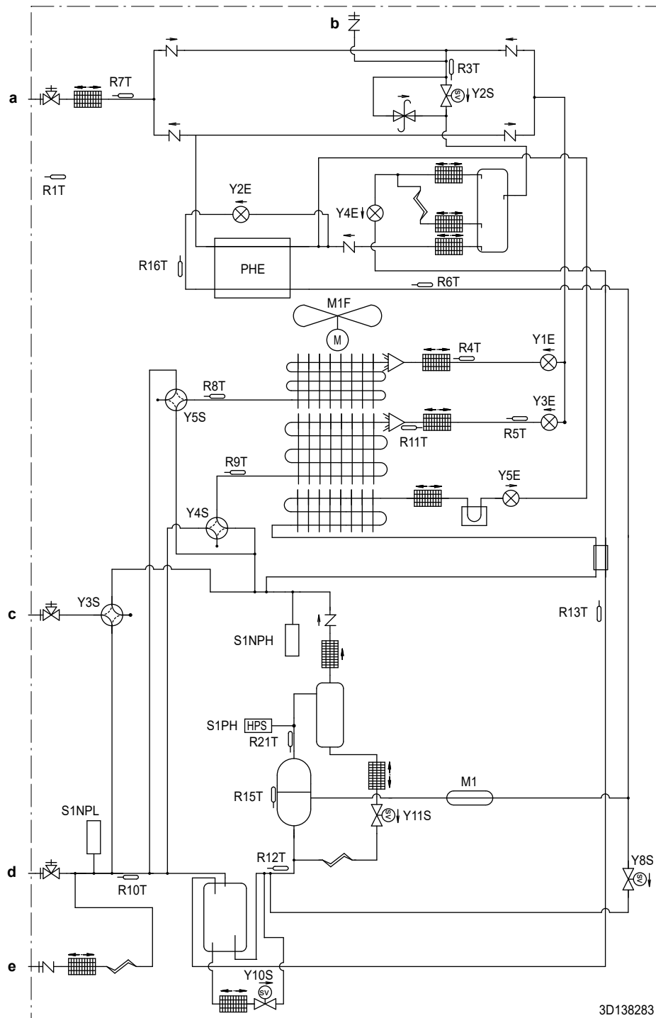
Leidingschema: 5~12 HP
