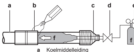
a Koelmiddelleiding
